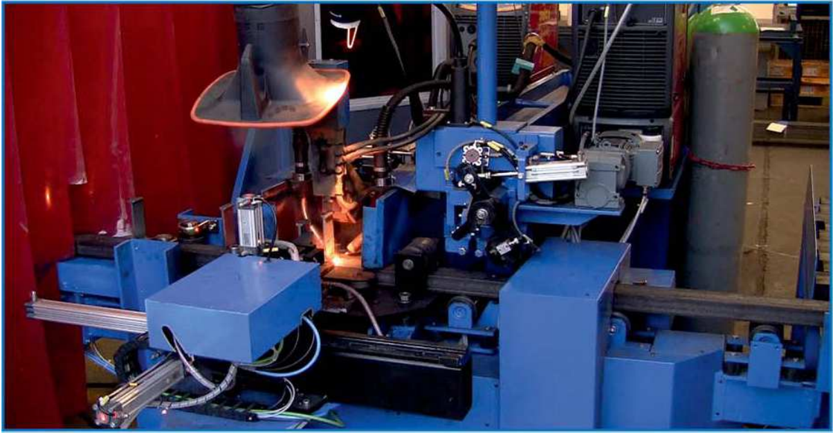
Automatizovano postrojenje za zavarivanje, izrađeno po zahtevu Kupca
